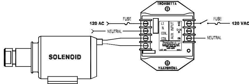
S500-A300 MODULE
